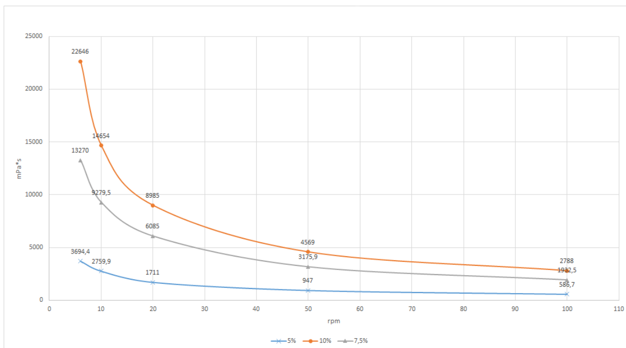
Rysunek 1. REOFELD 3UG - lepkość żelu wodnego w różnych stężeniach
