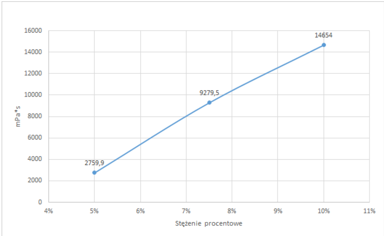
Rysunek 2. Zmiana lepkości żelu wodnego przy różnych stężeniach (R5/10)
